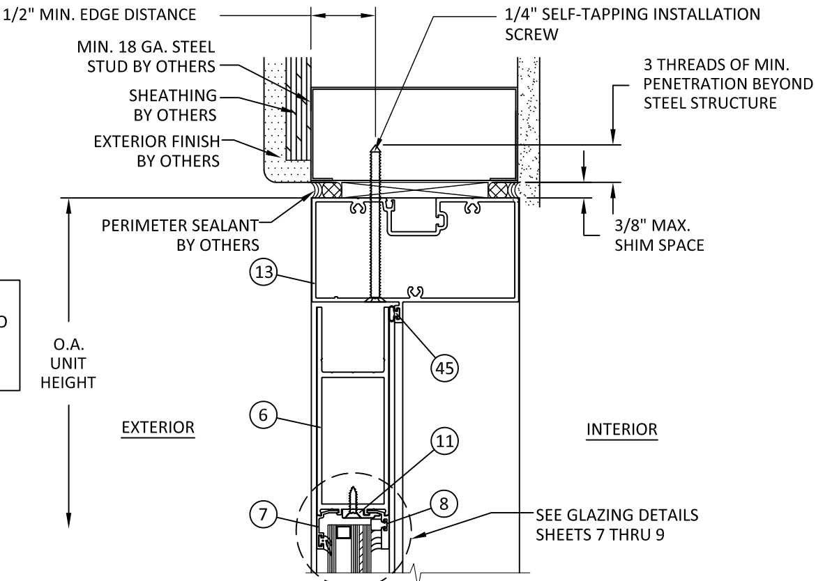
C 3 VERTICAL SECTION DOOR HEAD - STEEL STUD
