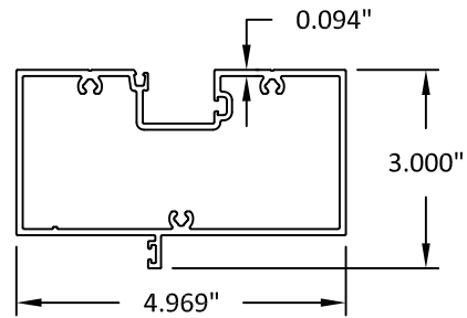
13 TRANSOM BAR (MONO)
