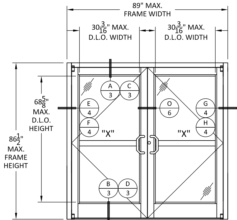
ELEVATION A DOUBLE DOOR
