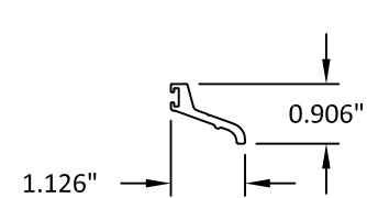
16 DOOR STOP
