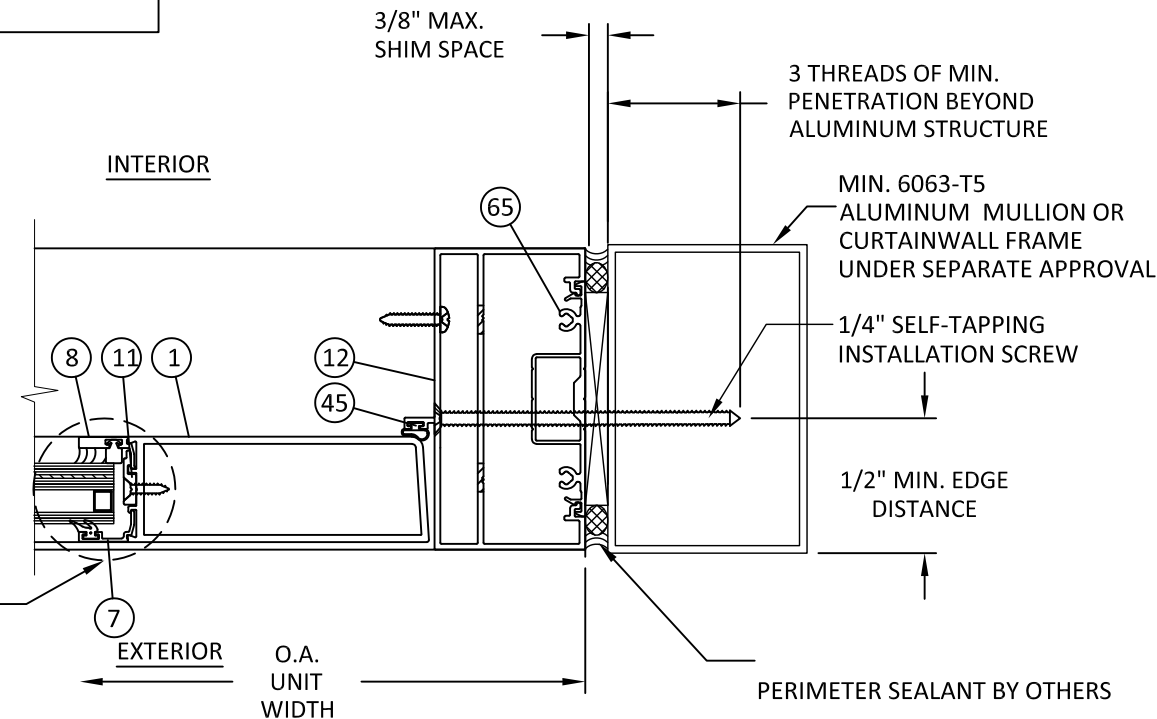
H 4 HORIZONTAL SECTION DOOR JAMB - ALUMINUM STUD
